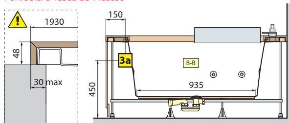
Particolare vasca ad incasso
